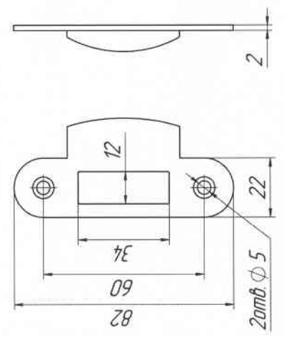
Ответная планка
