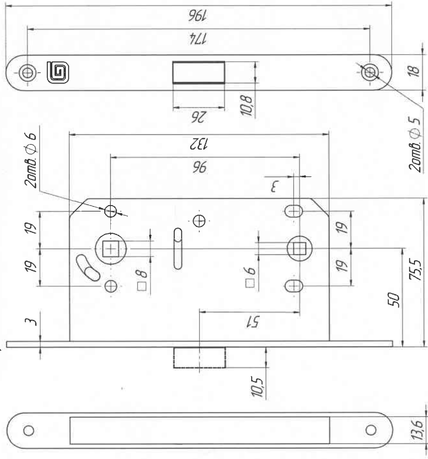
Защелка "SOFT 1 M" (ЗВМ.07.00)
